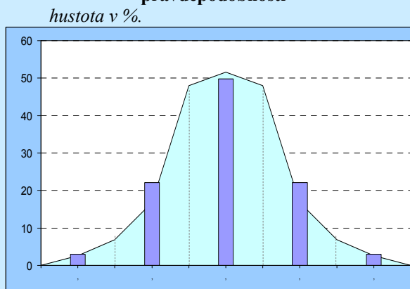
Graf C.1.2: Normální rozložení pravděpodobností
